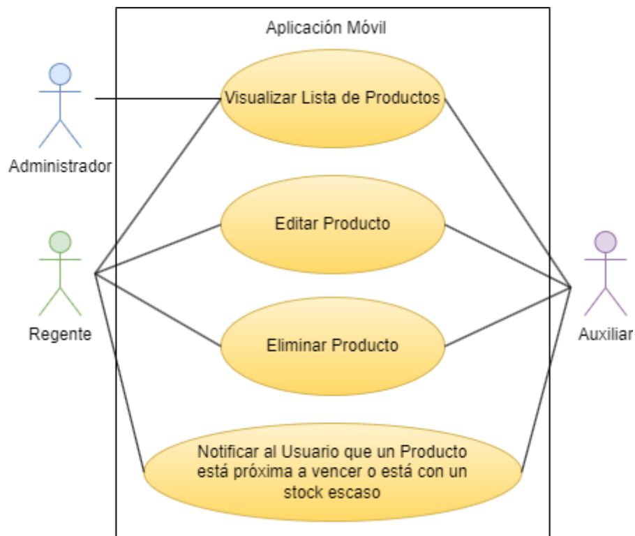
Figura 3.6. Diagrama de Casos de Uso de la Gestión de Stock .
