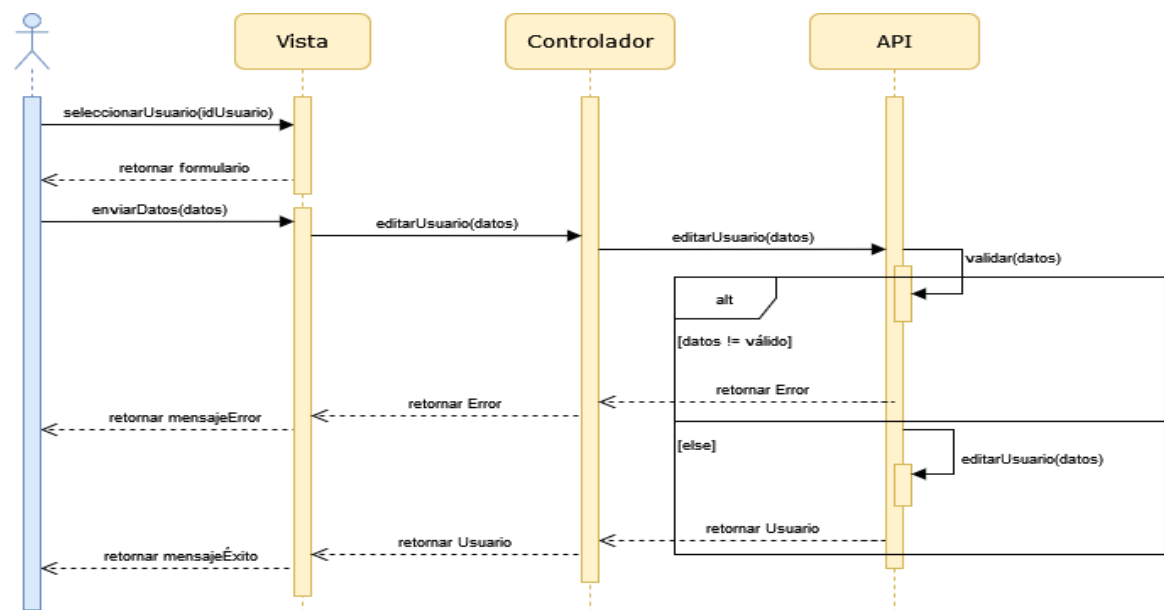
Figura 3.18. Diagrama de Secuencias de la Edición de Usuarios.
