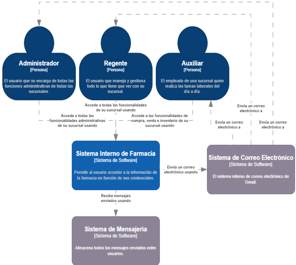
Figura 3.11. Diagrama de Contexto del Sistema de la Farmacia.
