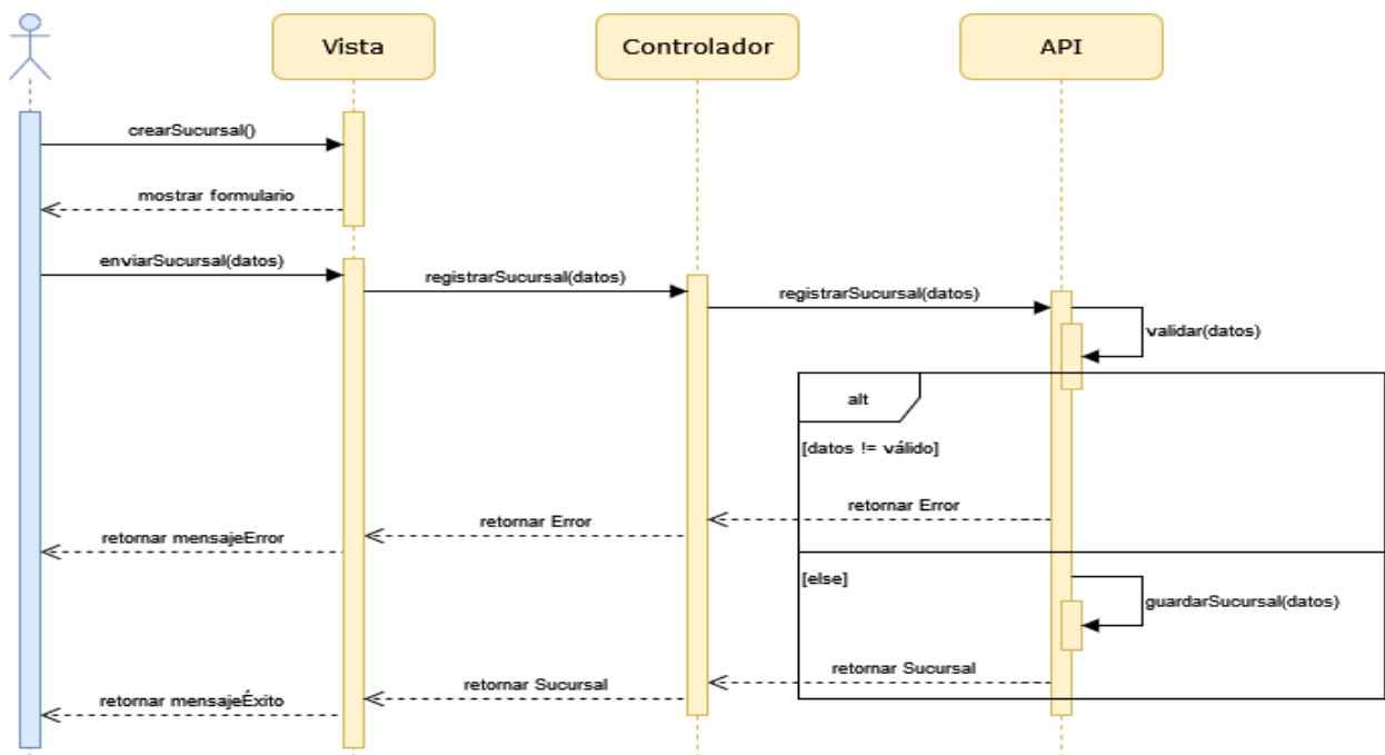
Figura 3.22. Diagrama de Secuencias del Registro de Sucursales.
