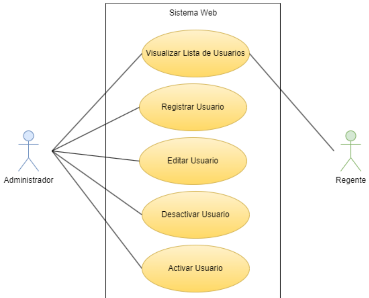
Figura 3.2. Diagrama de Casos de Uso de la Gestión de Administrador y Usuarios.
