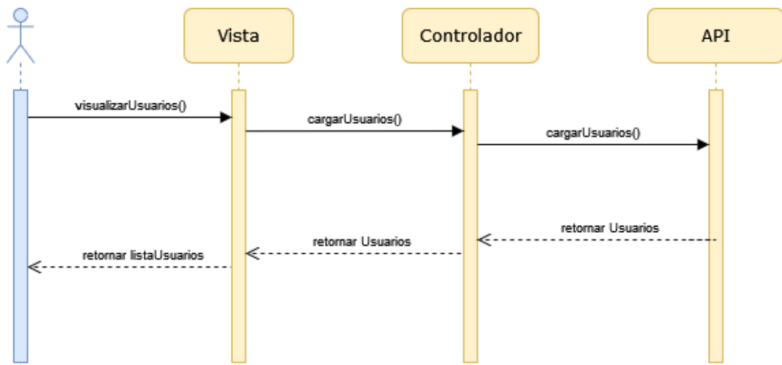
Figura 3.16. Diagrama de Secuencias de la Visualización de Lista de Usuarios.
