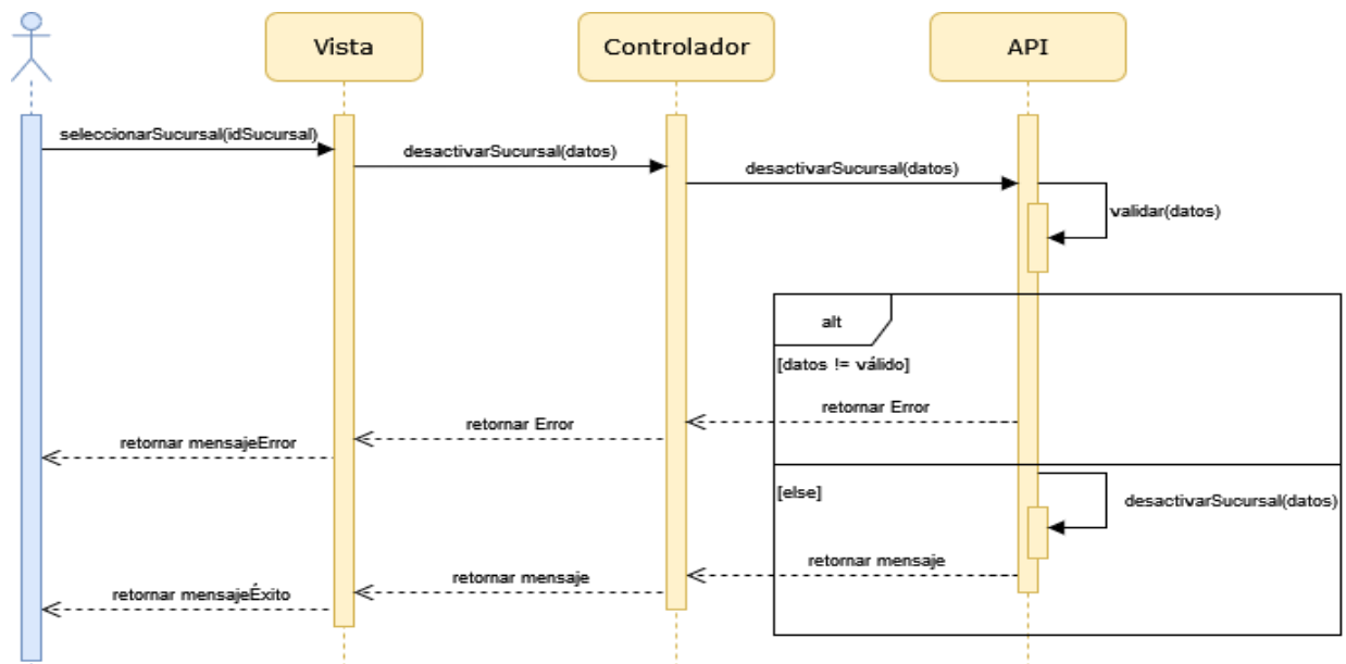
Figura 3.24. Diagrama de Secuencias de la Desactivación de Sucursales.
