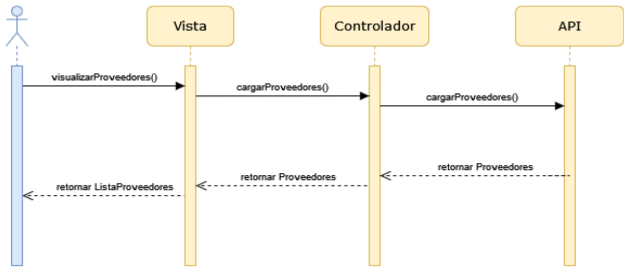
Figura 3.26. Diagrama de Secuencias de la Visualización de Lista de Proveedores.
