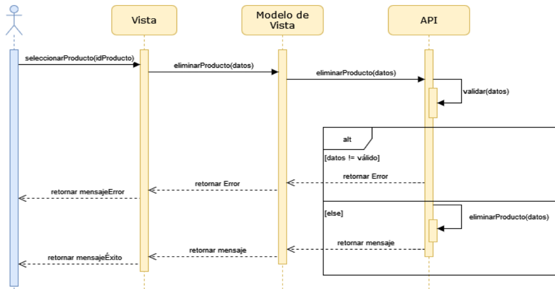
Figura 3.36. Diagrama de Secuencias de la Eliminación de Productos.
