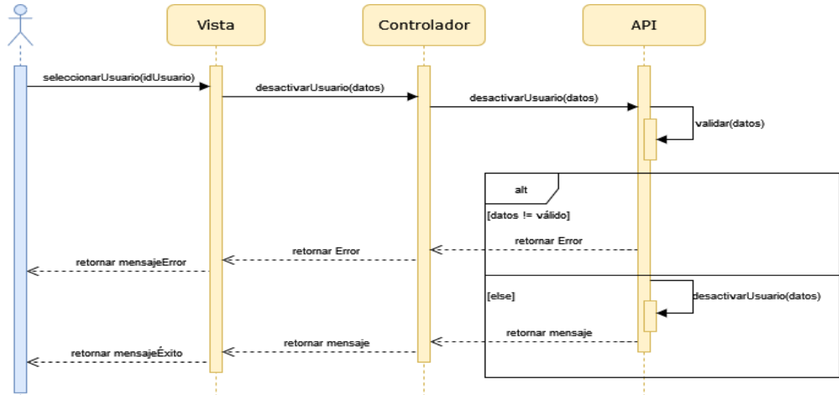
Figura 3.19. Diagrama de Secuencias de la Desactivación de Usuarios.
