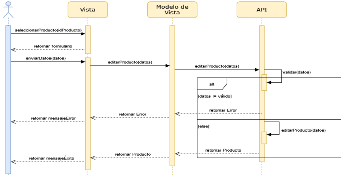
Figura 3.35. Diagrama de Secuencias de la Edición de Productos.
