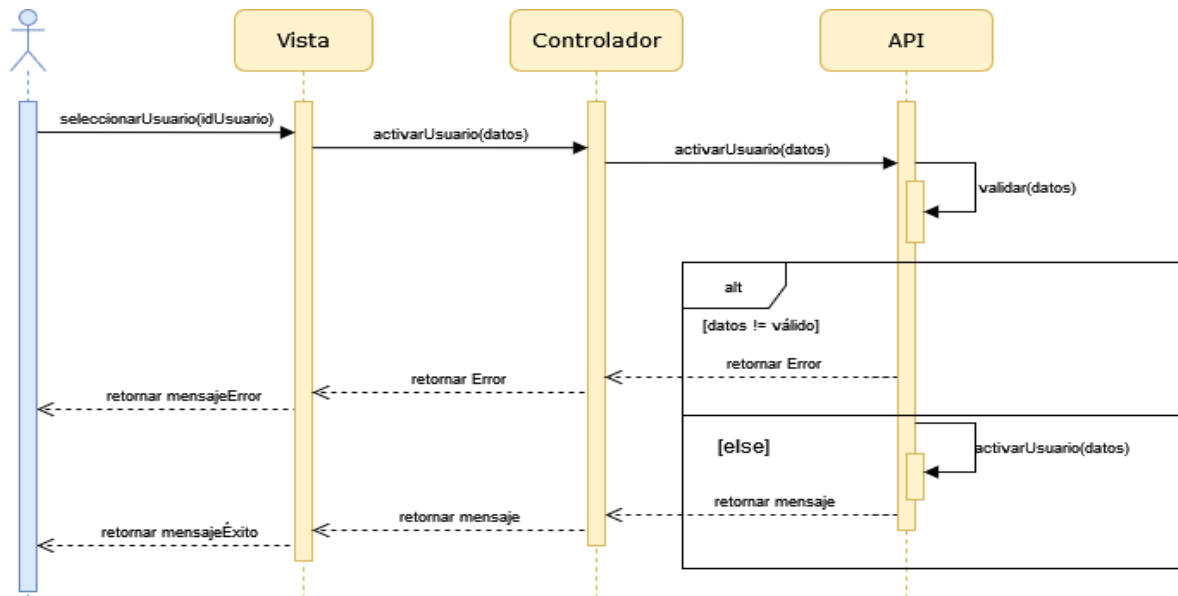
Figura 3.20. Diagrama de Secuencias de la Activación de Usuarios.
