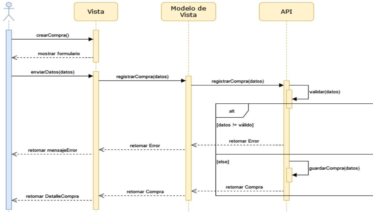
Figura 3.32. Diagrama de Secuencias del Registro de Compras.
