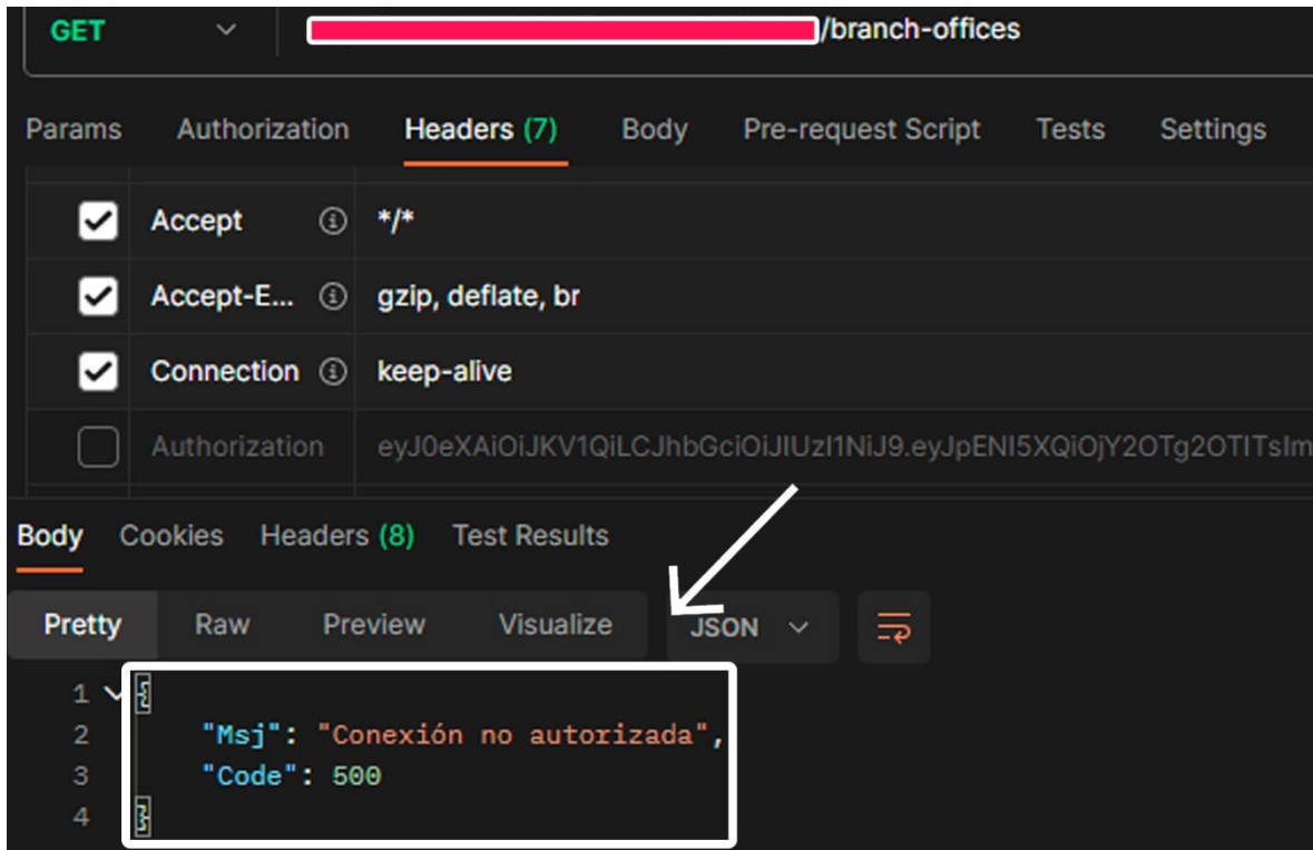
Figura 4.6. Consulta a la API sin el JWT (mediante Postman).
