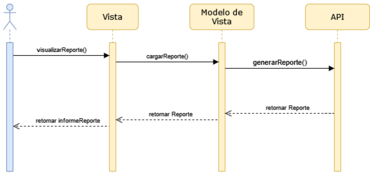
Figura 3.40. Diagrama de Secuencias de Generación de Reportes.
