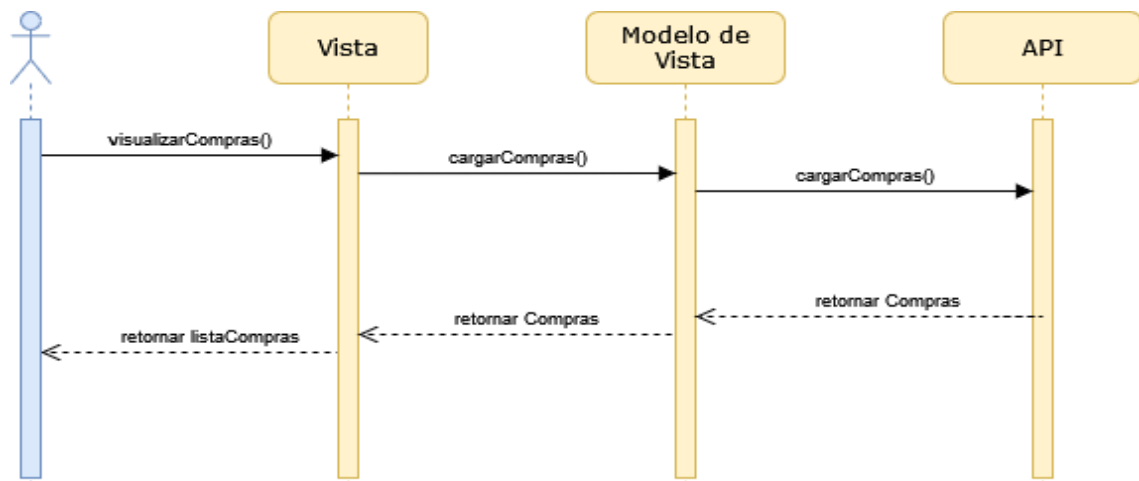
Figura 3.31. Diagrama de Secuencias de la Visualización de Lista de Compras.
