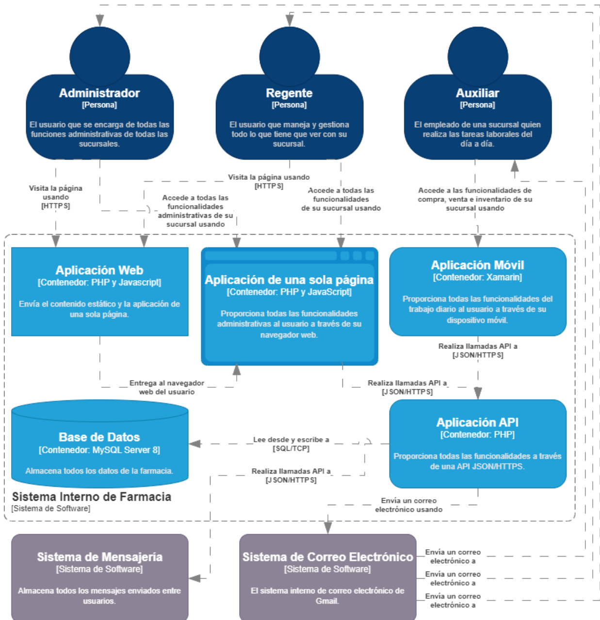
Figura 3.12. Diagrama del Contenedor del Sistema de la Farmacia.
